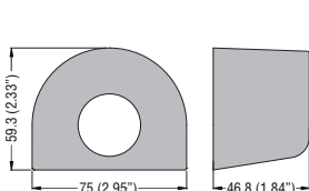
LPXAU159
