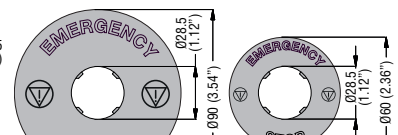
LPXAU112 LPXAU113
