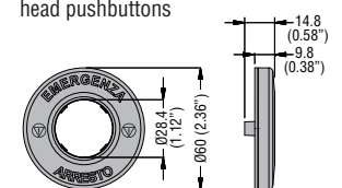
LPXDAU11...
