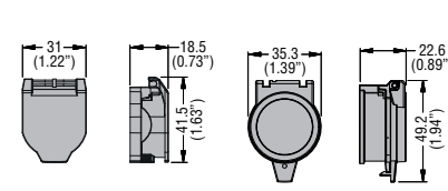
LPXAU170
