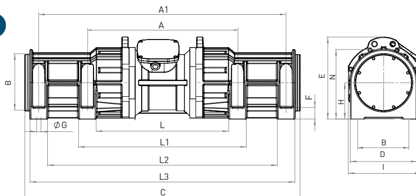
DIMENSIONI DI INGOMBRO (mm)
